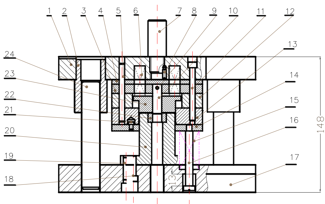
模具图
