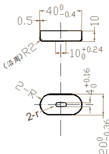
图一：冲压零件
