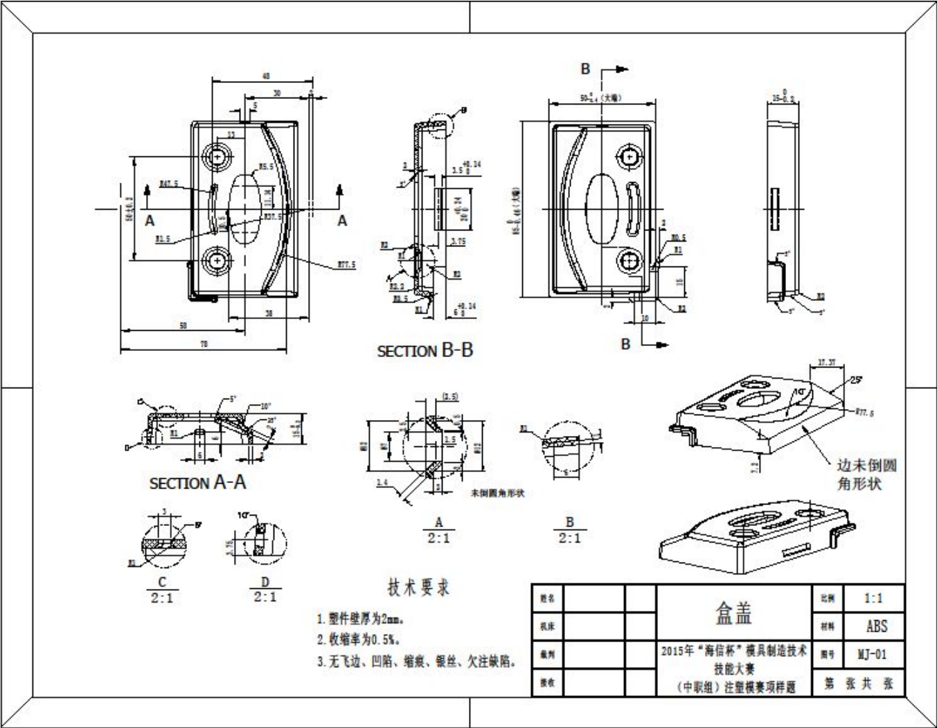
附图1：塑件制作图
