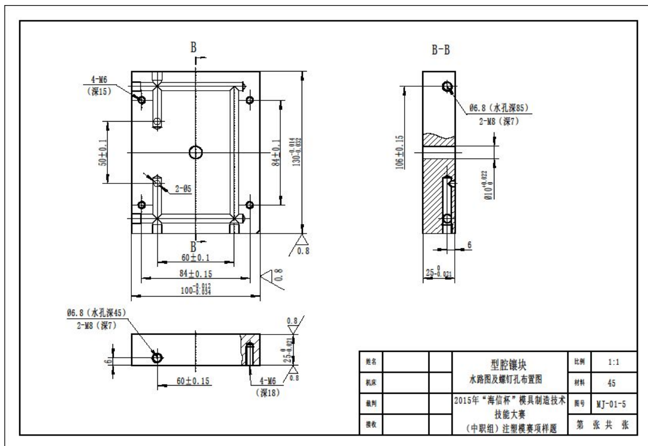
附图5：型腔镶块螺纹孔及水路布置图
