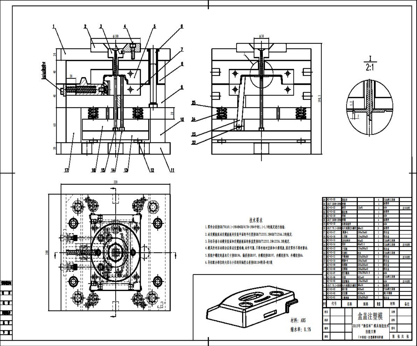
附图2：模具装配图
