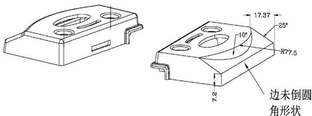
图一：塑料制品三维外形图
